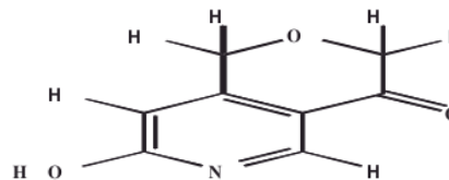
Gambar 1. 7-hidroksipiranopiridin-4-on
