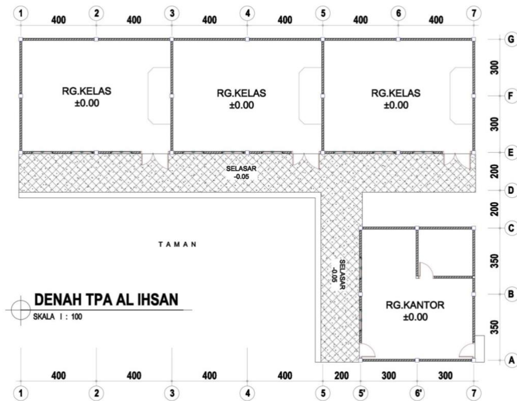
Gambar 3. Denah Bangunan TPA Al Ihsan Sumber: Hasil Tim Kegiatan Pengabdian, 2020
