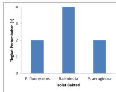
Gambar 8 Hasil uji kualitatif pertumbuhan bakteri pada limbah kilang yang mengandung amoniak.
