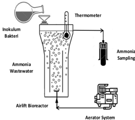
Gambar 4 Diagram skematik Bioreactor yang digunakan.
