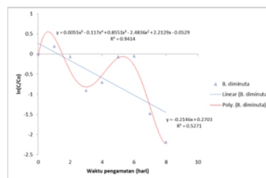
Gambar 10 Laju penurunan kadar amoniak.
