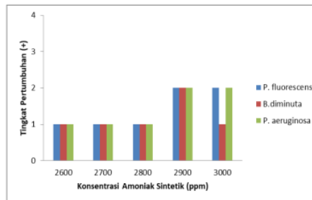
Gambar 8 Hasil uji kualitatif pertumbuhan bakteri pada amoniak sintetik.
