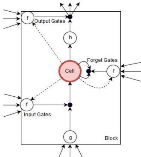
Gambar 4.14. Arsitektur LSTM
