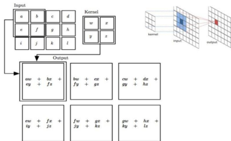
Gambar 4.3. Operasi Konvolusi
