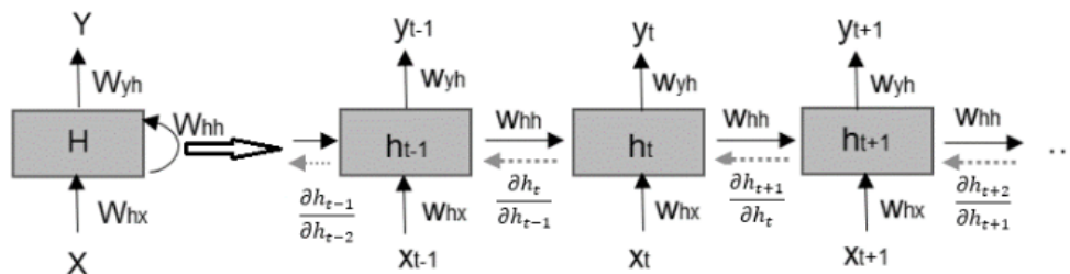
Gambar 4.12. Struktur RNN
