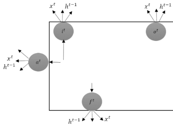
Gambar 4.21. Perubahan komputasi input dan gate pada backward pass
