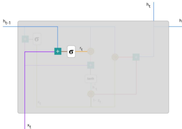
Gambar 4.23. Proses reset gate
