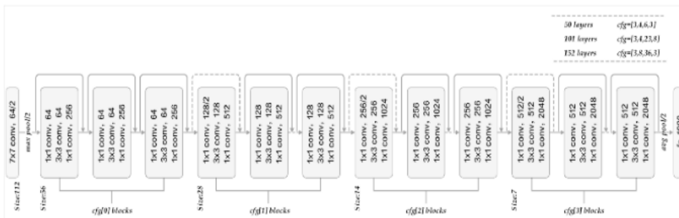
Gambar 4.9. Arsitektur ResNet (He et al., 2016)
