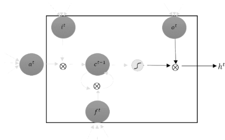
Gambar 4.18. Proses LSTM hingga menghasilkan output
