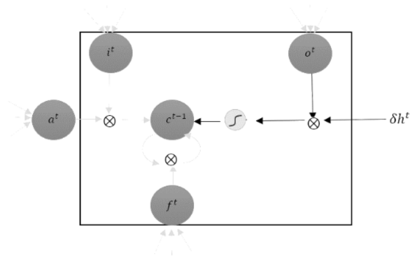
Gambar 4.19. Proses backward pass dari hasil keluaran forward pass
