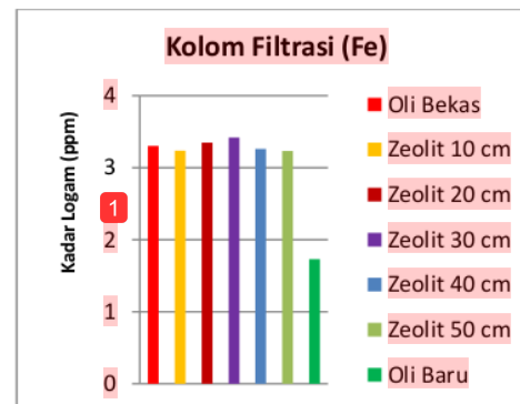
Gambar 2. Diagram Pengaruh Tinggi Kolom Filtrasi Zeolit Terhadap Logam Fe
