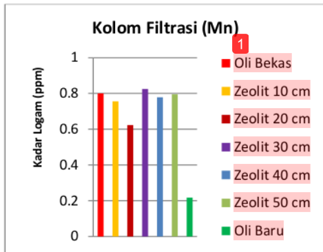
Gambar 3. Diagram Pengaruh Tinggi Kolom Filtrasi Zeolit Terhadap Logam Mn
