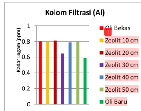
Gambar 1. Diagram Pengaruh Tinggi Kolom Filtrasi Zeolit Terhadap Logam Al
