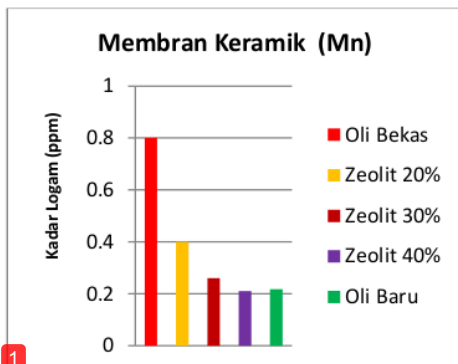
Gambar 8. Diagram Pengaruh Komposisi Zeolit Pada Membran Keramik Terhadap Kandungan Logam Mn
