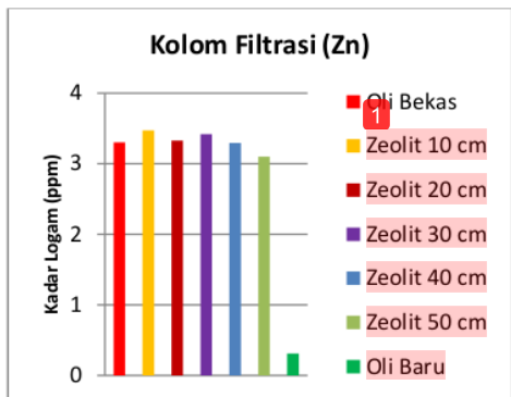
Gambar 4. Diagram Pengaruh Tinggi Kolom Filtrasi Zeolit Terhadap Logam Zn
