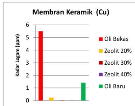
Gambar 10. Diagram Pengaruh Komposisi Zeolit Pada Membran Keramik Terhadap Kandungan Logam Cu
