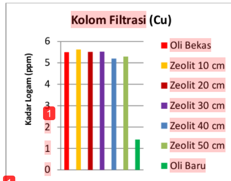
Gambar 5. Diagram Pengaruh Tinggi Kolom Filtrasi Zeolit Terhadap Logam Cu
