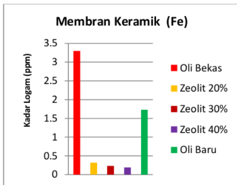
Gambar 7. Diagram Pengaruh Komposisi Zeolit Pada Membran Keramik Terhadap Kandungan Logam Fe
