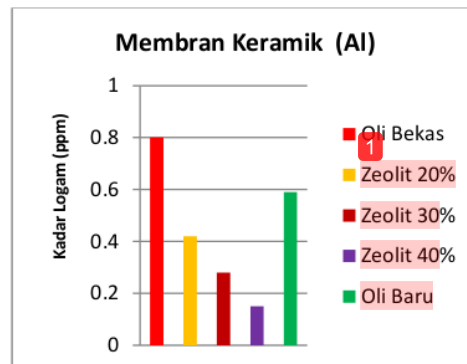
Gambar 6. Diagram Pengaruh Komposisi Zeolit Pada Membran Keramik Terhadap Kandungan Logam Al
