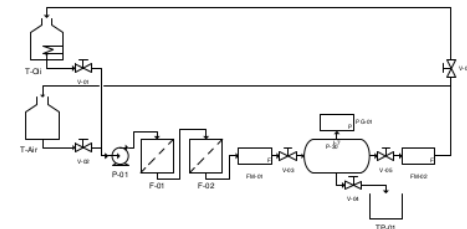
Gambar 2. Proses Membran Keramik
