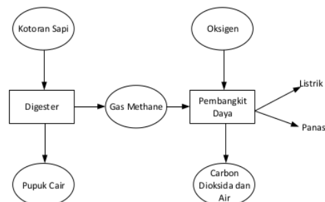
Gambar 5. Skema Pembangkit Listrik Biogas
