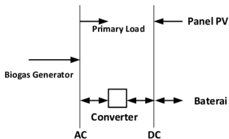
Gambar 6. Skema Sistem Teknologi Hibrid Matahari dan Biogas
