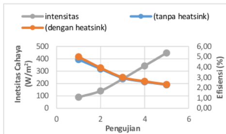
Gambar 5 Perbandingan efisiensi FV1 dan FV2 terhadap intensitas cahaya.
