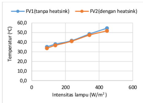
Gambar 4 Kenaikan temperatur permukaan panel photovoltaic terhadap intensitas cahaya.
