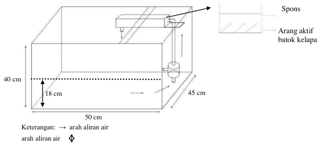
Gambar 1. Desain sistem resirkulasi dengan filterisasi
