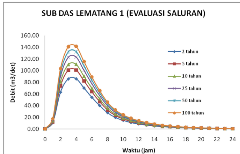
Gambar 5. HSS di hilir saluran di sub DAS Lematang-1
