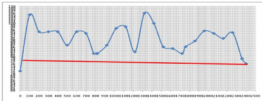
Gambar 7. (a) Jalur normalisasi sungai; (b) Kemiringan dasar saluran
