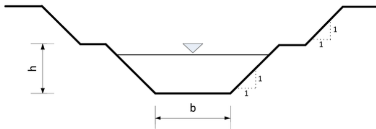
Gambar 6. Tipikal saluran terbuka
