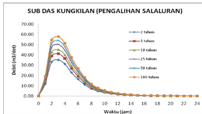
Gambar 4. HSS di pengalihan saluran pada sub DAS Kungkulan
