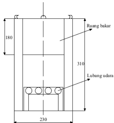
Gambar. 2 Kompor sisa kayu atau sekam
