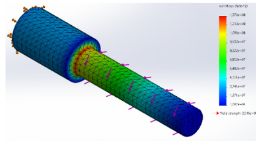
Gambar 5. Hasil Simulasi Pengujian Variasi Terhadap Tegangan Von Mises
