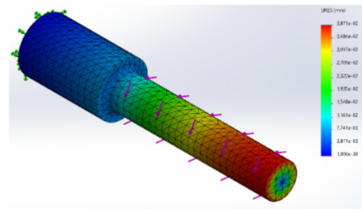
Gambar 6. Hasil Simulasi Pengujian Variasi Terhadap Displacement
