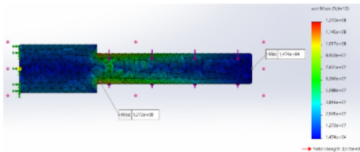
Gambar 3. Hasil Simulasi Investigasi Terhadap Tegangan Von Mises
