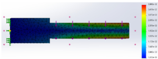
Gambar 4. Hasil Simulasi Investigasi Terhadap Displacement
