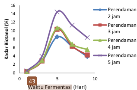
Gambar 4. Grafik Pengaruh Waktu Fermentasi 75 gram Sekam Padi terhadap Kadar Bioetanol yang Dihasilkan
