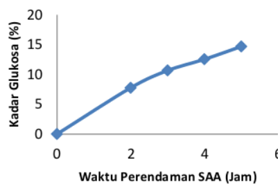
Gambar 2. Grafik Pengaruh Waktu Perendaman 75 gram Sekam Padi dalam 300 ml Larutan Amonia 15% pada Proses Pretreatment terhadap Kadar Glukosa
