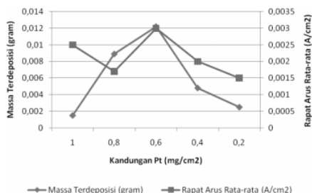
GAMBAR 2: Massa Terdeposisi dan Rapat Arus Rata-rata pada perbandingan massa Pt bervariasi untuk Elektroda Pt/C
