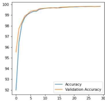
Gambar 3 Grafik Akurasi Model U-Net
