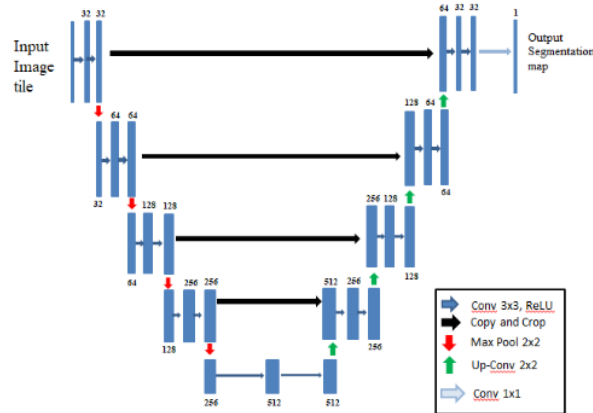
Gambar 1 Arsitektur U-Net
