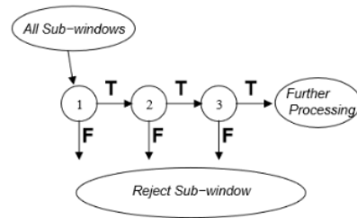
1 Fig. 3. Cascade classifier.
