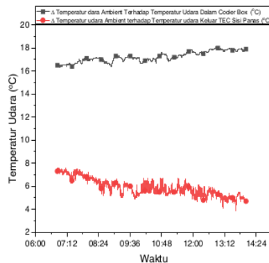
Gambar 4. Beda temperatur ambient dan temperatur udara dalam dan ke luar kotak pendingin terhadap waktu
