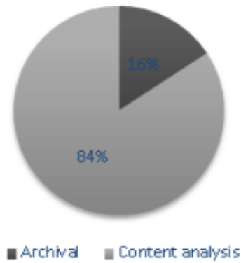
Gambar 3. Metode Riset
