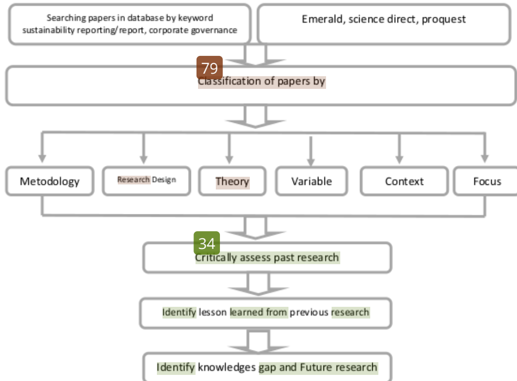
Gambar 1. Kerangka Penelitian
