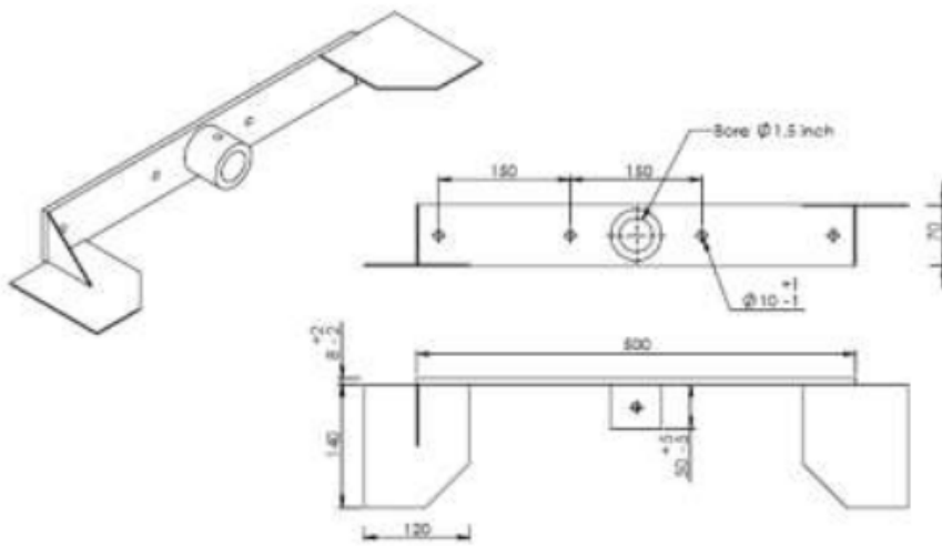
Pisau Pemotong 2-b
