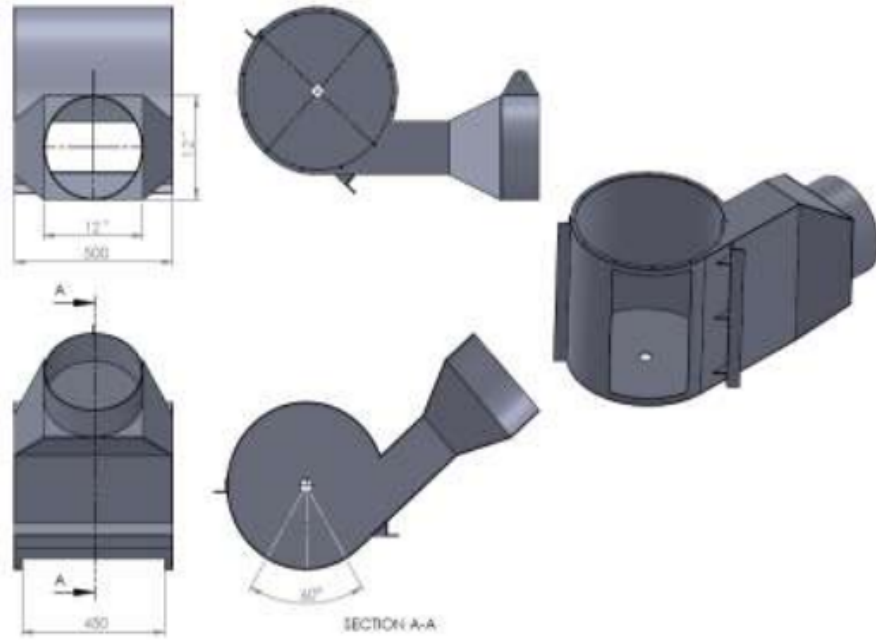
Tutup Turbin Air-2
