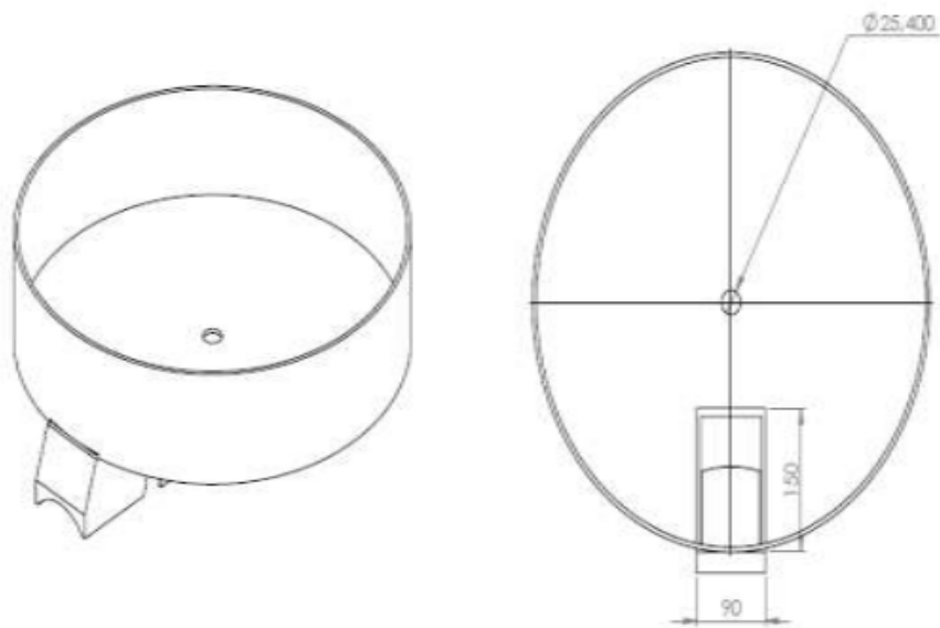
Bak Penutup (atas)
