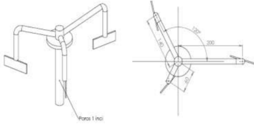
Pengaduk
