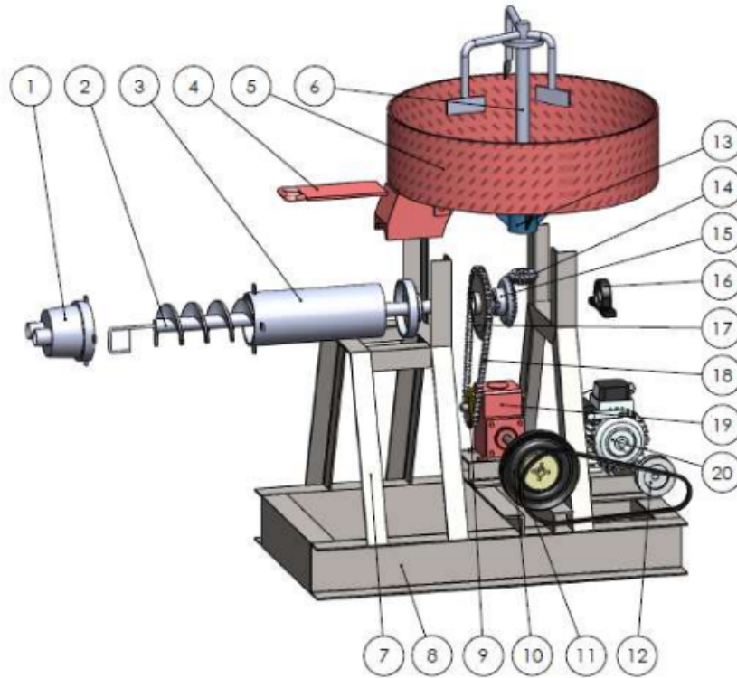
Gambar 5.1 Alat pencetak biobriket multi guna
