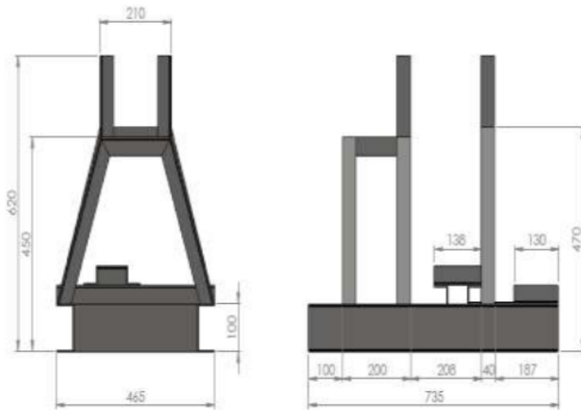
Dudukan Rangka
