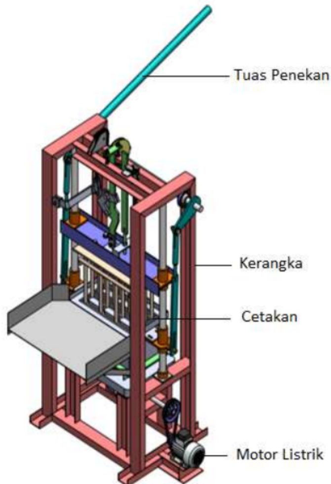
Gambar 5.2 Alat pencetak batako multi guna
