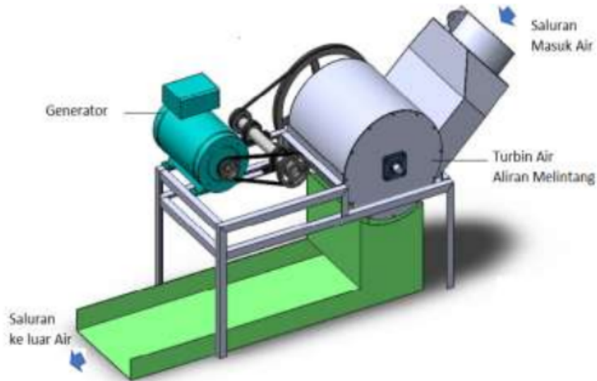
Gambar 7.1 Turbin air aliran melintang
