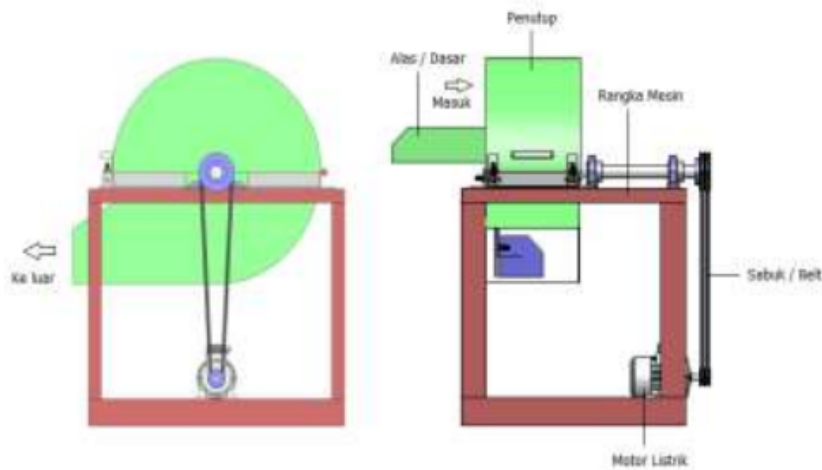
Gambar 6.1 Alat Pencacah Pakan Ternak
