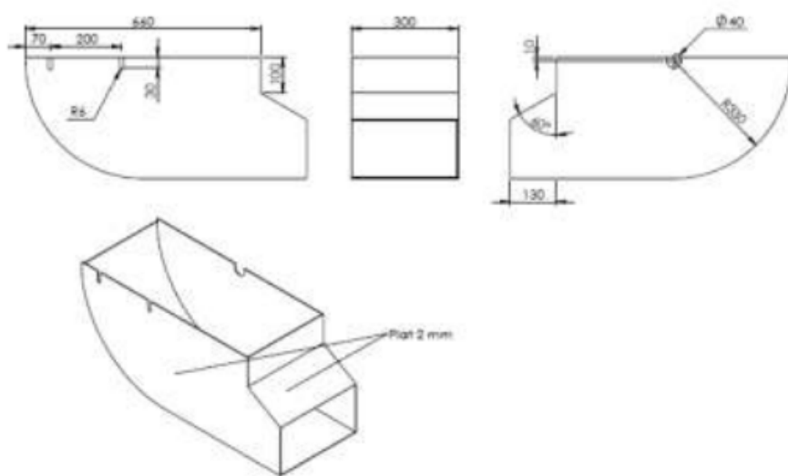
Penutup Bawah
