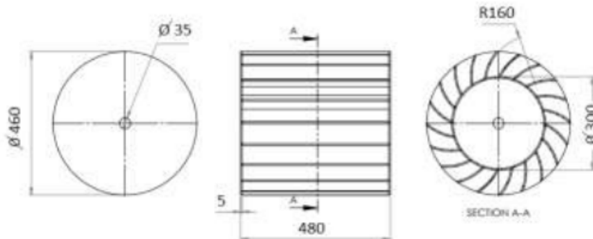
Gambar 7.2 Sudu gerak
