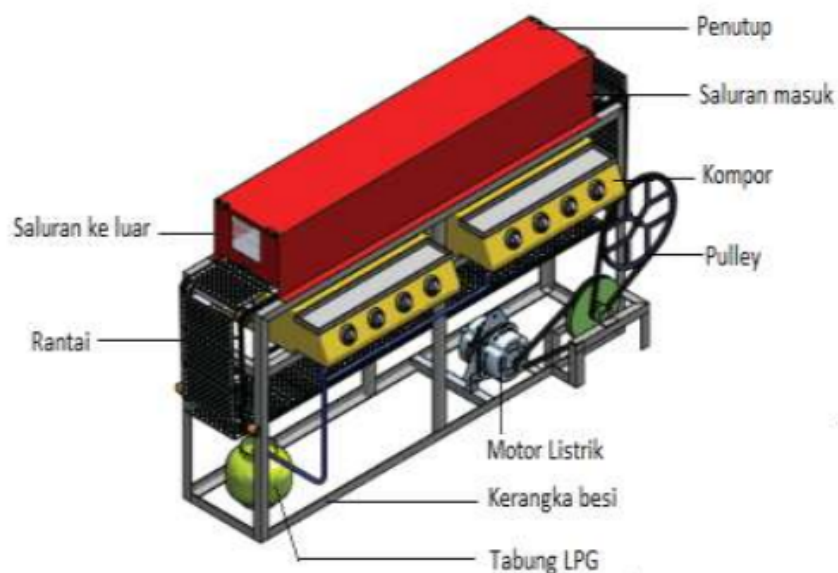
Gambar 2.2 Pemanggang teknologi infrared burner
