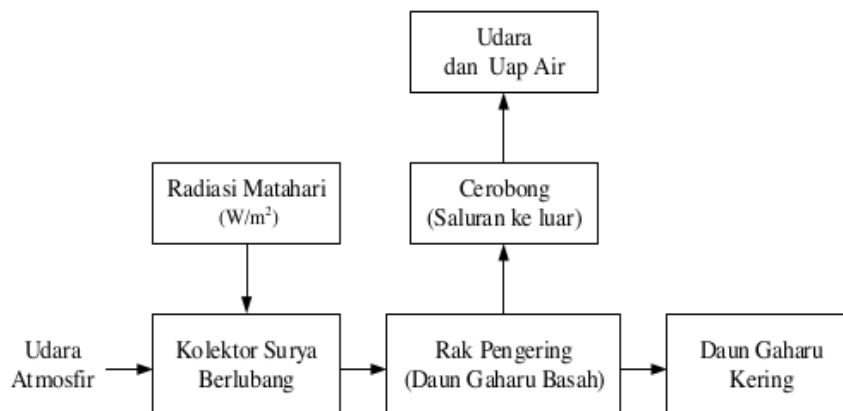
Gambar 3.4 Skema proses pengeringan daun gaharu
