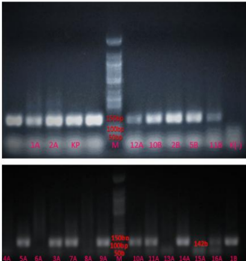
Gambar 3. Hasil elektroforesis menggunakan primer Mitin (142bp) Marker = DNA ladder 50bp.
