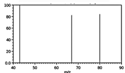
6,9,12-Octadecatrien-1-ol Anticancer
