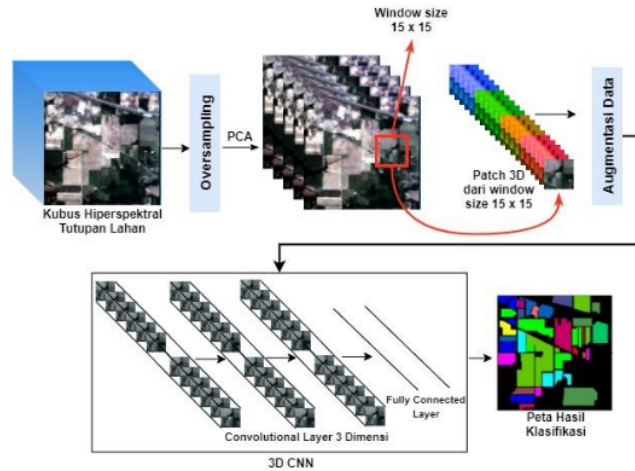
1 Gambar 4. Ilustrasi Proses Klasifikasi Pada Penelitian Ini
