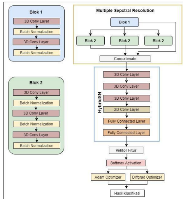
Gambar 8. Usulan Kombinasi MSR dan HybridSN
