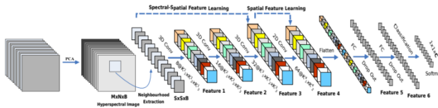
Gambar 5. Arsitektur HybridSN [15]
