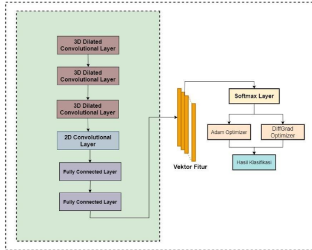
Gambar 9. Usulan Kombinasi Metode SDC dan HybridSN
