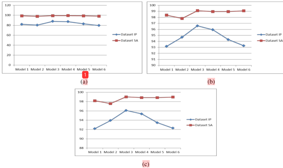
Gambar 10. Perbandingan Akurasi AA, OA dan Kappa Dari Masing-Masing Model Yang Diuji Pada Dataset IP dan SA
