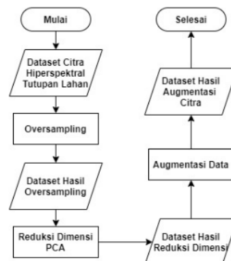
Gambar 3. Tahapan Praproses
