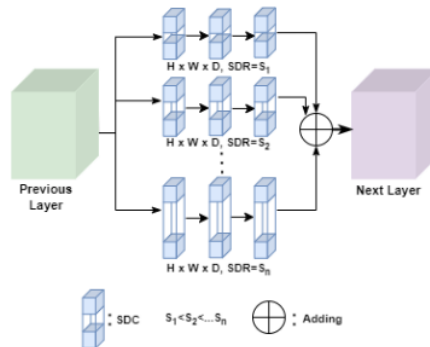
Gambar 6. Arsitektur MSR [16]
