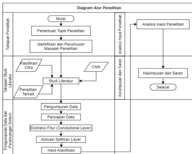
Gambar 1. Tahapan Penelitian
