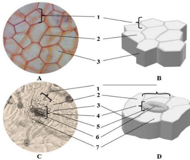
Gambar 10. Representasi 3D Daun Bunga Jepun ( Nerium oleander ); Permukaan adaksial (A= 2D; B= 3D); Permukaan abaksial (C= 2D; D= 3D); 1. Sel Epidermis; 2. Sitoplasma; 3. Dinding Sel; 4. Stomata; 5. Sel Penutup; 6. Celah Stomata; 7. Sel Tetangga.
