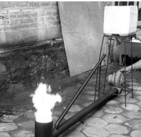
Gambar 6. Penyalan Kompor oli bekas
