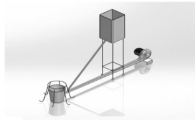
Gambar 2. Disain 3D Kompor oli bekas
