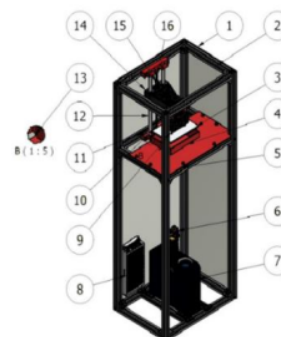
Gambar 1 Desain alat yang disosialisasikan
