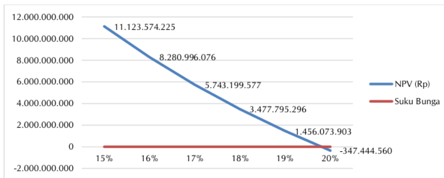
Gambar 5. Grafik perhitungan nilai NPV
