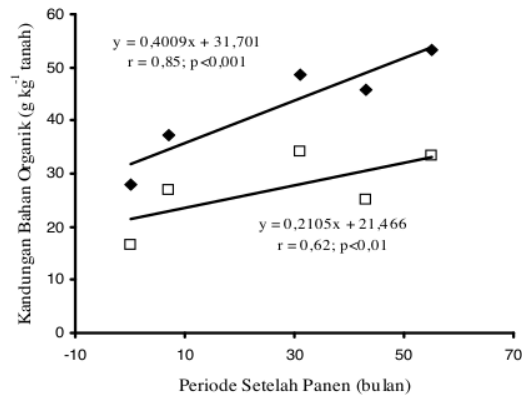
Gambar 1. Hubungan periode setelah panen dengan kandungan bahan organik tanah lahan Acacia mangium pada kedalaman 0-10 cm (◆) dan 10-20 cm (□).
