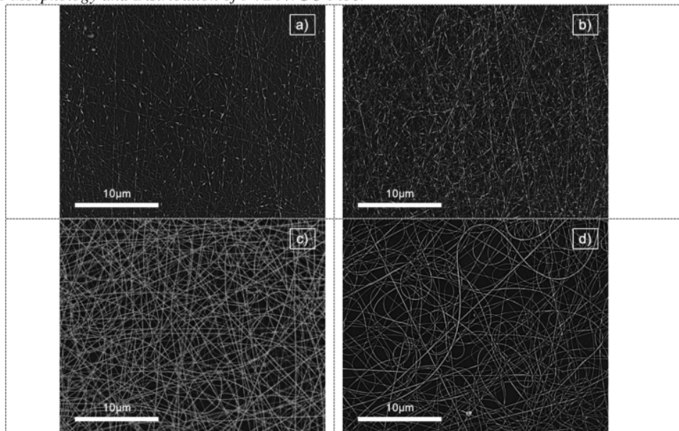
Figure 1. Morphology of PVDF/carbon (a) FPC 1, (b) FPC 2, (c) FPC 3 dan (d) FPC4 fiber.
