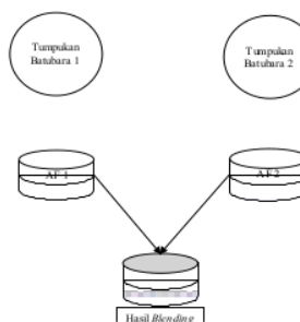
Gambar 2. Metode Dua Conveyor
