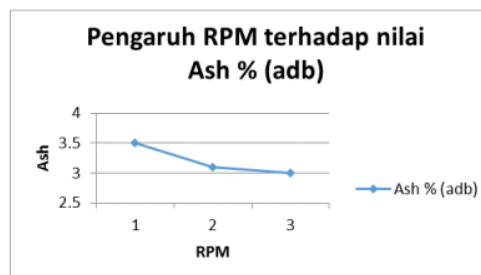
Gambar 7. Pengaruh kandungan abu terhadap RPM
