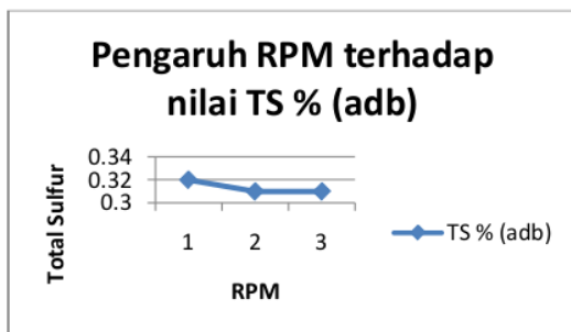
Gambar 8. Pengaruh kandungan total Sulphur terhadap RPM
