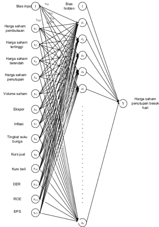
Gambar 1. Arsitektur Jaringan Backpropagation
