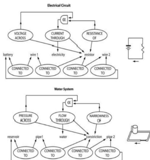
Gambar 1. Peta Struktur untuk rangkaian listrik dan sistem air, diadaptasi dari Gentner (Sumber : Podolefsky, 2004)
