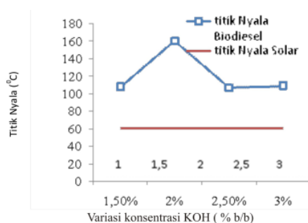
GAMBAR 3: Hubungan Variasi konsentrasi KOH dengan Titik Nyala
