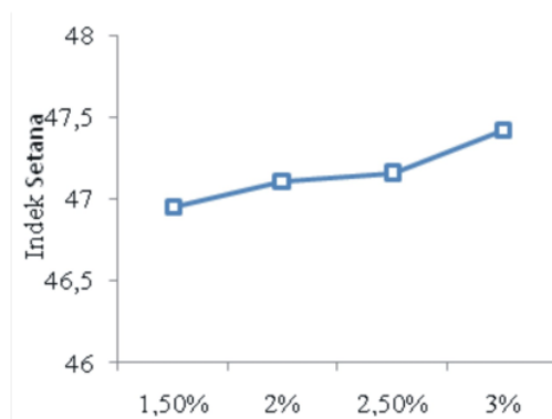
GAMBAR 2: Hubungan Variasi konsentrasi KOH dengan Indek Setana
