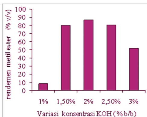
GAMBAR 1: Grafik perolehan metil ester dengan variasi konsentrasi KOH
