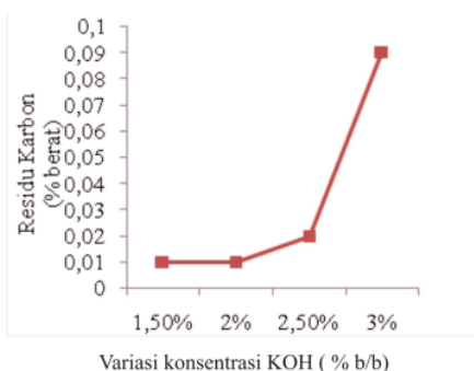
GAMBAR 5: Hubungan Variasi konsentrasi KOH dengan Residu Karbon
