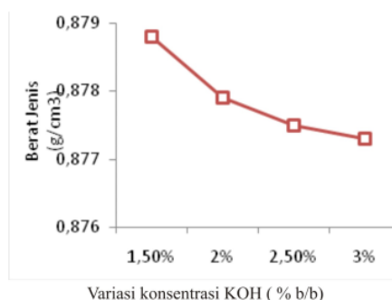
GAMBAR 6: Hubungan Variasi konsentrasi KOH dengan Berat Jenis
