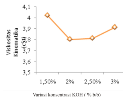
GAMBAR 4: Hubungan Variasi konsentrasi KOH dengan Viskositas Kinematika
