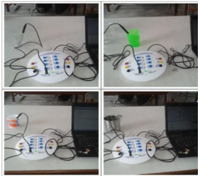
Gambar 5. Pengukuran suhu untuk keempat wadah
