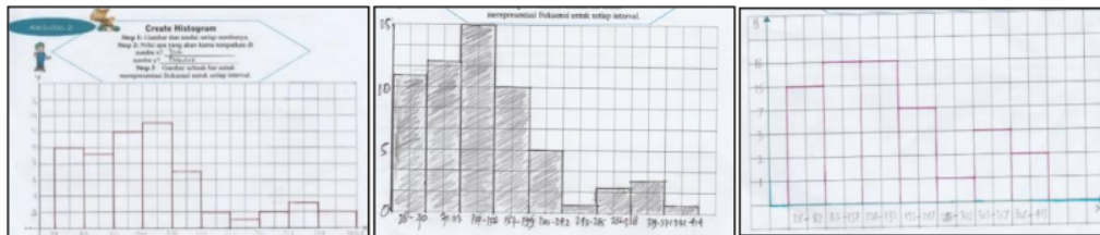
Gambar 6. Histogram 10 kelas
