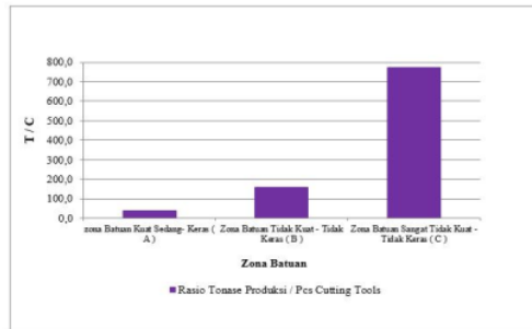
Gambar 8. Grafik perbandingan tonase produksi vs konsumsi cutting tools di 3 zona batuan
