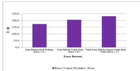
Gambar 7. Grafik perbandingan tonase produksi vs hour unit di 3 zona batuan
