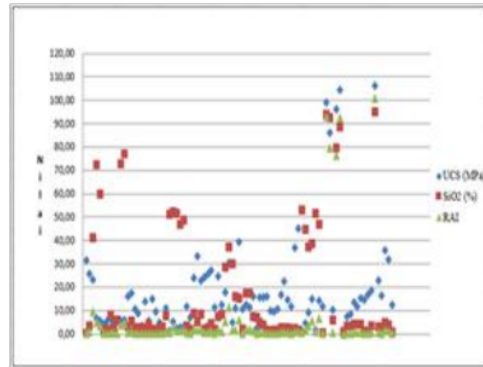
Gambar 4. Grafik nilai UCS – SiO 2 – RAI sampel pengeboran dan permukaan
