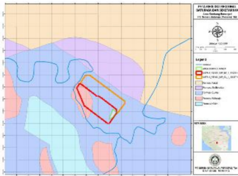
Gambar 2. Peta geologi regional semen Baturaja.
