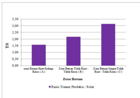
Gambar 9. Grafik perbandingan tonase produksi vs konsumsi bahan bakar di 3 zona batuan
