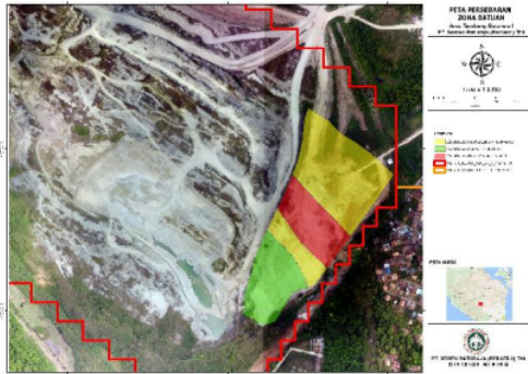
Gambar 5. Peta penyebaran batugamping dengan nodule silika di lokasi penelitian
