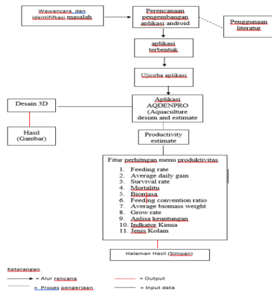
Gambar 1. Alur penelitian pengembangan aplikasi AQDENPRO
