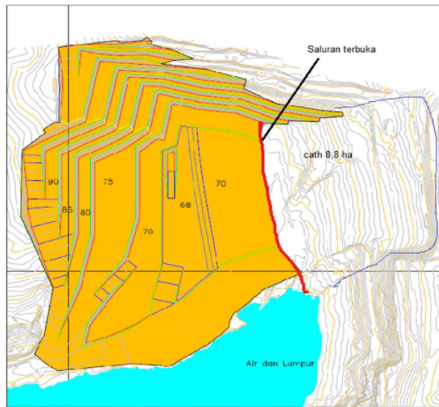
Gambar 4. Posisi Saluran Terbuka
