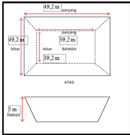
Gambar 2. Dimensi Sump Rencana
