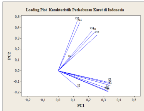
Gambar 2 Loading plot karakteristik perkebunan karet
