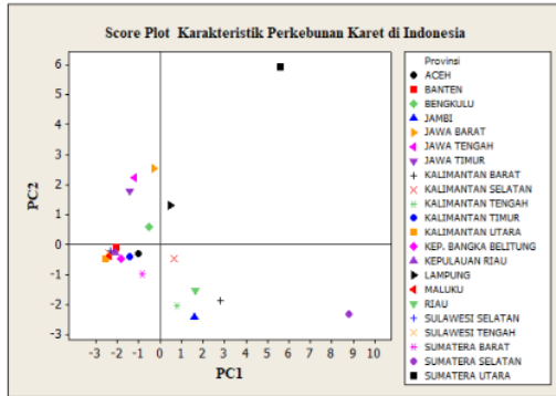
Gambar 3 Skor komponen provinsi
