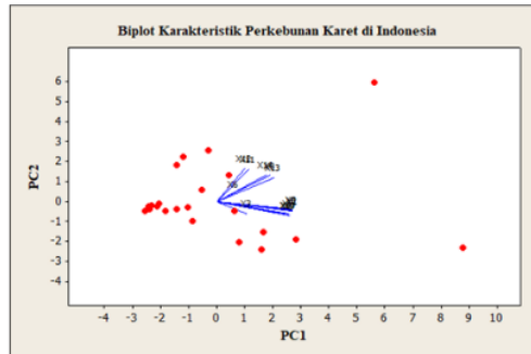
Gambar 1 Biplot Karakteristik Perkebunan Karet
