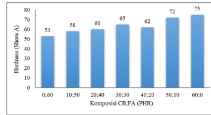
Gambar 1. Pengaruh Variasi Jumlah Filler Terhadap Hardness Vulkanisat
