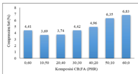
Gambar 4. Pengaruh Variasi Jumlah Filler Terhadap Compression Set Vulkanisat
