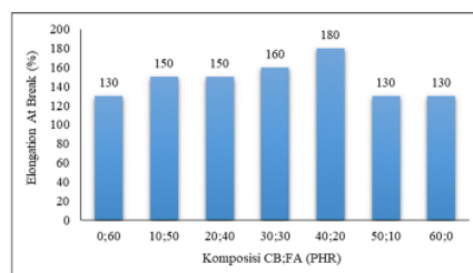
Gambar 3. Pengaruh Variasi Jumlah Filler Terhadap Elongation At Break Vulkanisat
