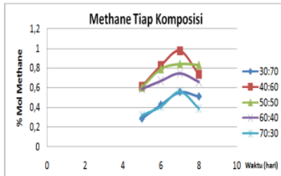
Gambar 1 Grafik Hubungan Antara Persentase Mol Methane Terhadap Waktu Menggunakan Starter EnviroSolve
