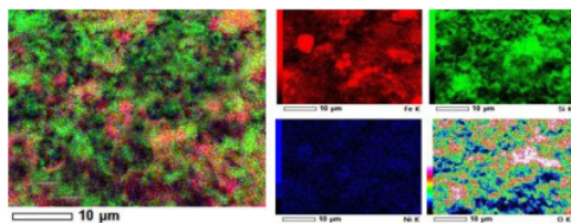
Figure 5. SEM Mapping of Fe 3 O 4 /SiO 2 /NiO
