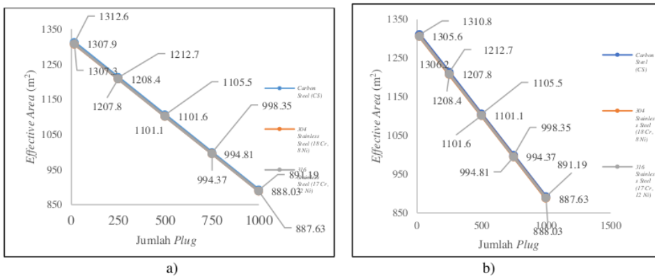
Gambar 7. Effective Area : a) 127-CA dan b) 127-CB
