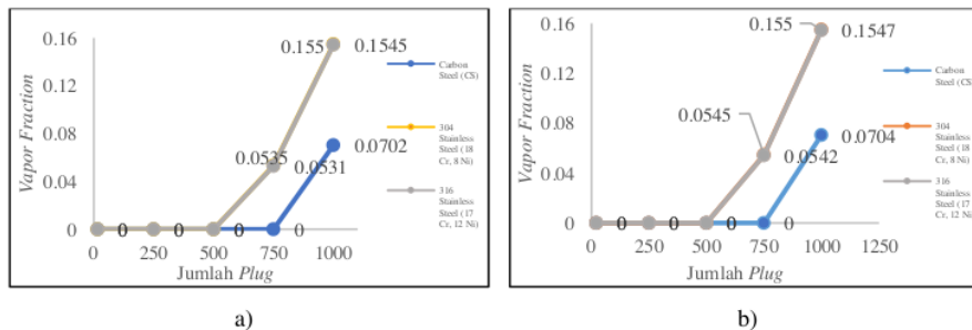
Gambar 4. Vapor Fraction Keluaran Amonia: a) 127-CA dan b) 127-CB
