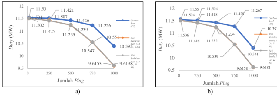
Gambar 6. Duty : a) 127-CA dan b) 127-CB
