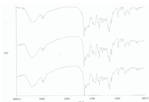
GAMBAR 4: Perbandingan spektrum inframerah senyawa hasil isolasi dengan senyawa morusin
