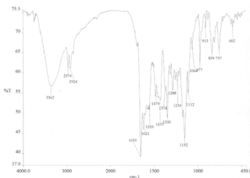
GAMBAR 3: Spektrum inframerah senyawa hasil isolasi
