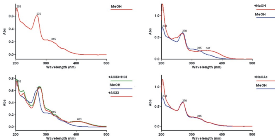
GAMBAR 2: Spektrum ultraviolet senyawa hasil isolasi
