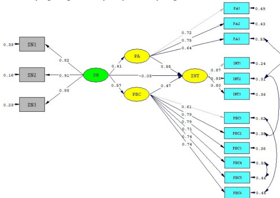
Gambar 2. Hasil Estimasi Parameter Full Model Struktural
