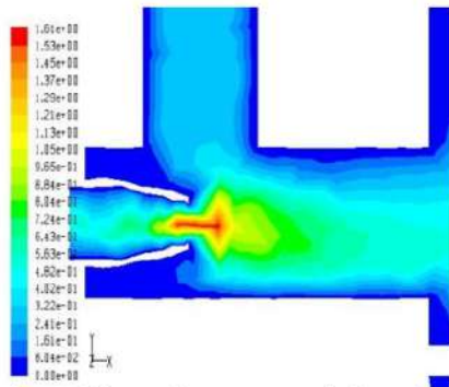
Gambar 7. Kontur Kecepatan pada Daerah nozel pada NXP-3
