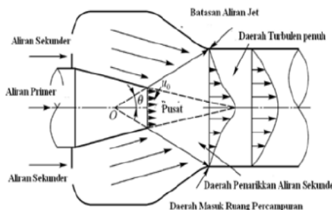
(c) Posisi keluaran Nozel menjauhi titik 0 (arah negatif)
