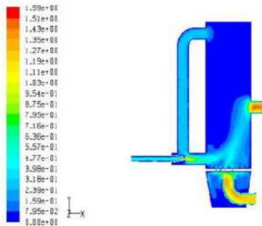
Gambar 6. Kontur kecepatan (m/s) Aliran Udara dalam Reaktor dengan Saluran Menggunakan ejektor
