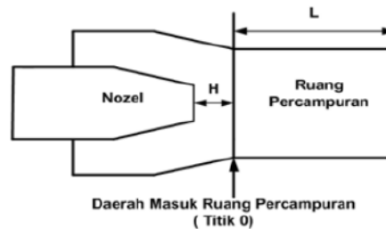
(a) Jarak Keluaran Nozel terhadap titik 0 (H)
