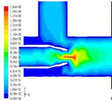
Gambar 8. Kontur Kecepatan pada Daerah nozel pada NXP 0
