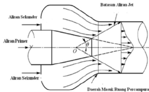
(b) Posisi Keluaran Nozel (H) mendekati titik 0 (arah positif)
