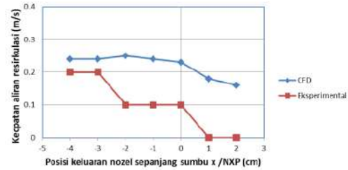
Gambar 10. Perbandingan CFD dan Eksperimen untuk kecepatan resirkulasi (m/s)
