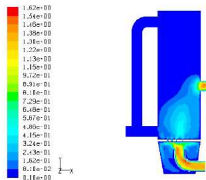
Gambar 5. Kontur Kecepatan (m/s) Aliran Udara dalam Reaktor dengan Saluran Resirkulasi tanpa Ejektor
