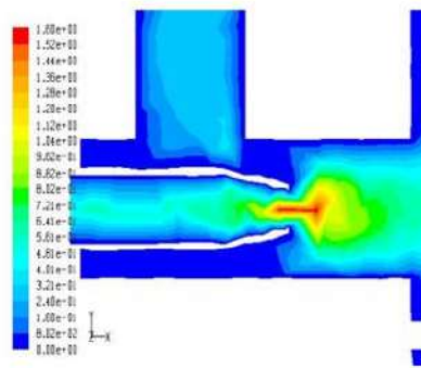
Gambar 9. Kontur Kecepatan pada Daerah Nozel pada NXP +2
