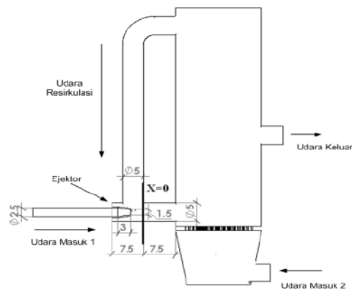
Gambar 1. Model Reaktor dan Ejektor (semua ukuran dalam cm)
