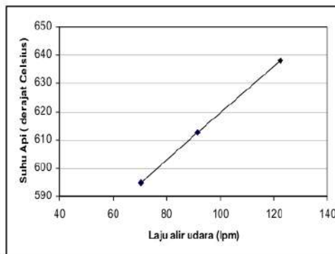
Gambar 7. Laju Aliran Udara vs Suhu Api
