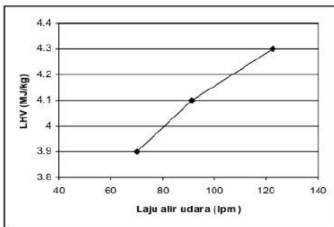
Gambar 5. Laju Aliran Udara vs LHV Gas
