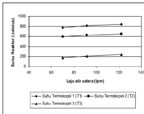
Gambar 3. Laju Aliran Udara vs Suhu Reaktor
