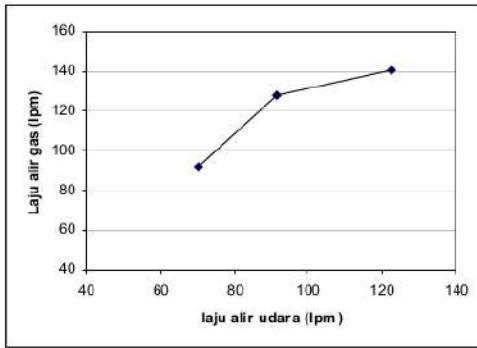
Gambar 4. Laju Aliran Udara vs Laju Aliran Gas yang Dihasilkan
