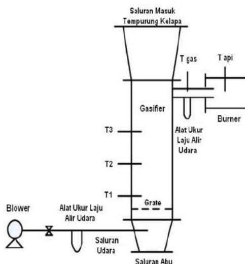
Gambar 1. Skema Set-up Eksperimen
