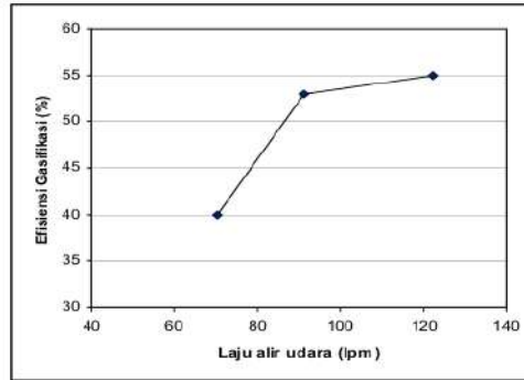
Gambar 6. Laju Aliran Udara vs Efisiensi Gasifikasi
