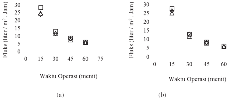
Gambar 3. Fluks pada berbagai variasi waktu operasi untuk filter dengan komposisi : a) tanah liat 72,5%, zeolit 25% dan serbuk besi 2,5 %; b) tanah liat 77,5%, zeolit 20% dan serbuk besi 2,5 % , □: P= 15,3 psi, ◻: P= 19,3 psi, ◊: P=23,3 psi)
