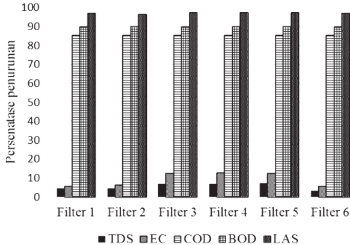
Gambar 4. Persentase penurunan parameter air limbah laundry
