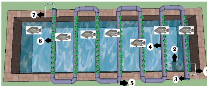
Gambar 1. Skema akuaponik.
