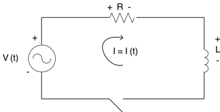
Gambar 1 Rangkaian RL
