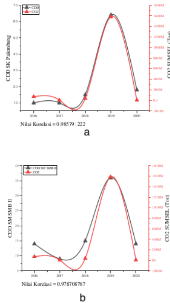
Gambar 1. Grafik hubungan antara CDD (a) SK Palembang dan (b) SM SMB II dengan GRK (Co2).
