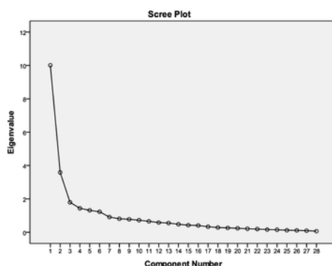
Gambar 1: Hasil Scree Plot 28komponen (Sumber: Analisis, 2017)
